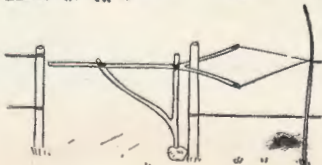
Svinglaage.
