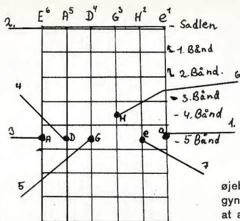
FIGUR 2 Diagrammet angiver, hvorledes guitaren stemmes
